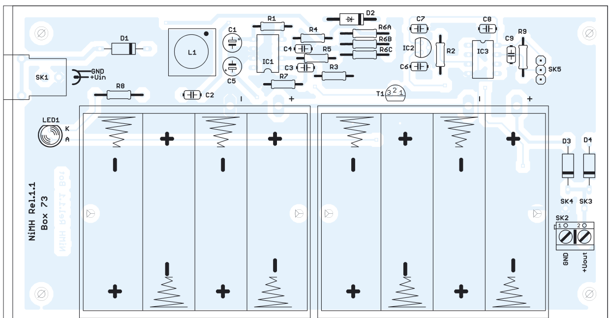
Bild 5: Die Spule L1 ist das einzige SMD-Bau- element. Als restliche Bauteile kommen bei der Bestückung nur bedrahtete Versionen zum Einsatz.
