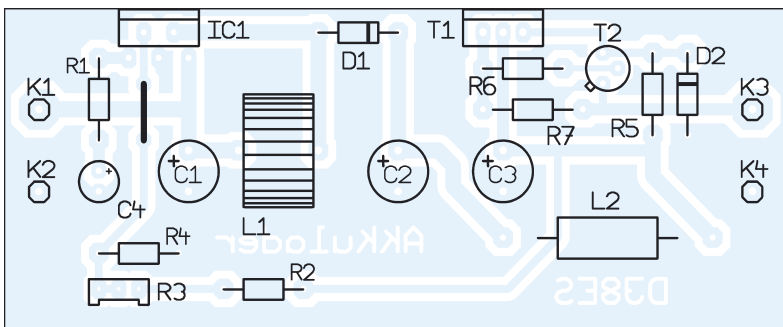
Bild 5: Bestückung erfolgt von der bis auf die Freisenkungen noch voll kaschierierten Seite aus.
