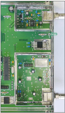
Auch mit betriebsfertiger Platine zu beziehen: FA-Netzwerktester
