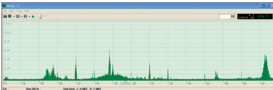
Bild 3: Der Screenshot von Rocky zeigt den Bereich von 133 bis 147 kHz. Deutlich sind (v. r. n. l.) DDH47 (Deutscher Wetterdienst), DCF39 Burg, ein Amateurfunksignal auf 137 kHz und ein weiterer kommerzieller Sender bei 135 kHz zu erkennen. Foto und Screenshot: DK1KQ
